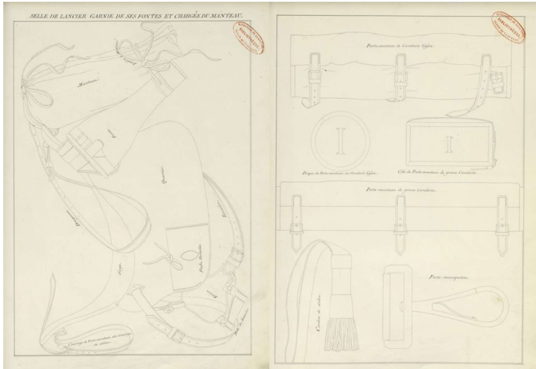
Tablice pokazujące siodło lansjerów oraz mantelzak lekkiej kawalerii, wg. Dessins faisant suite au règlement sur l'habillement , t. III, SHAT, MA 10872/A1J25.
