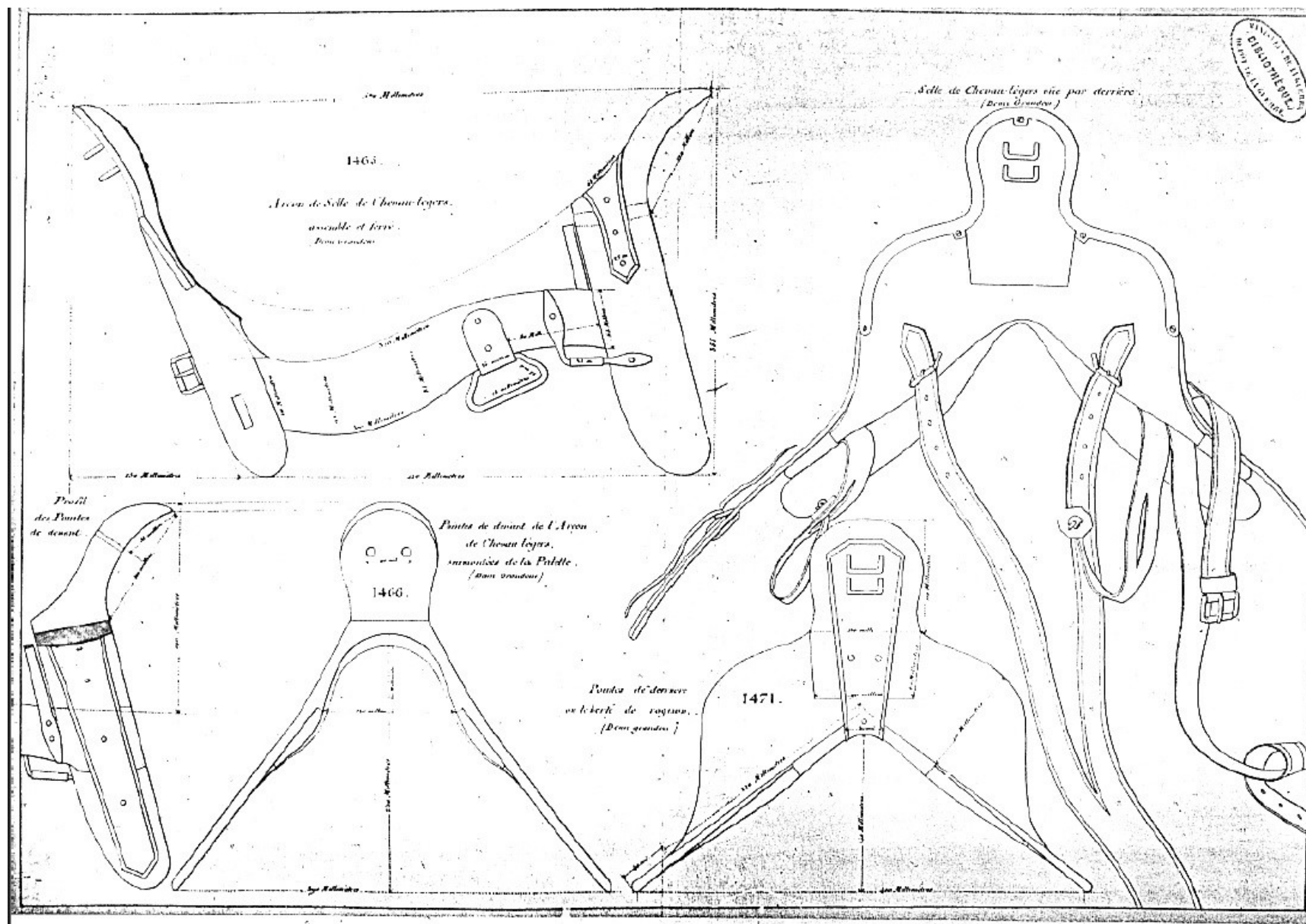
Tablica pokazujące detale siodła szwoleżerów (nr 1463, 1466, 1471), wg. Dessins Faisant .
